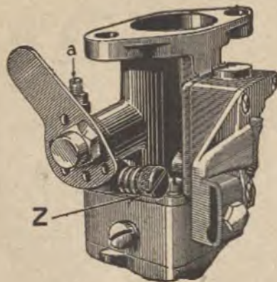
Abb. 6 Drosselklappenhebel mit Leerlaufregulierschraube Z und Öffnungsbegrenzungsschraube a.
