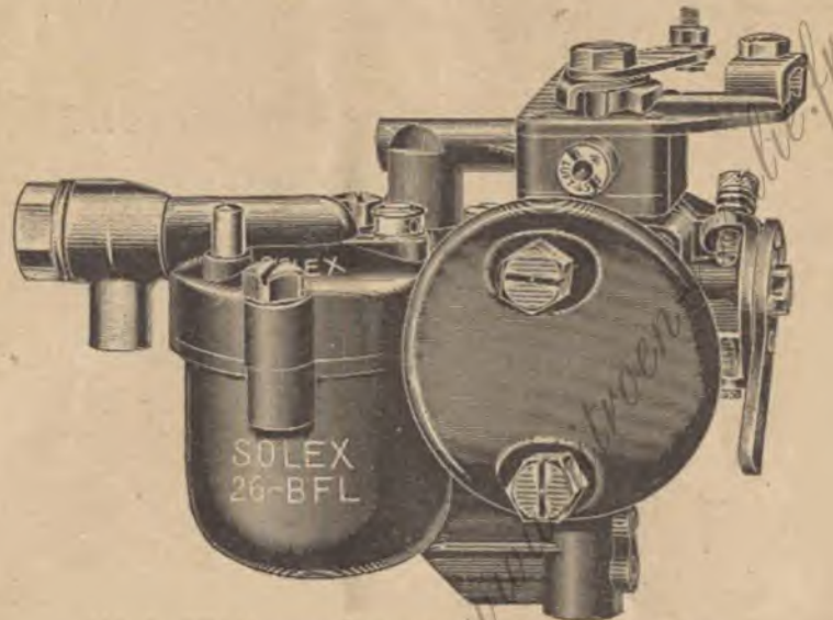
Abb. 2. BFH-Vergaser mit automatischer Startvorrichtung Horizontale Anordnung
